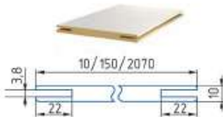
Добор телескопический/ прямой (МДФ) Размер: 10/150/2070
